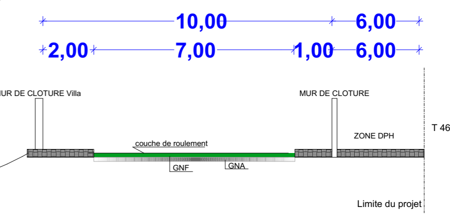
COUPE A-A
